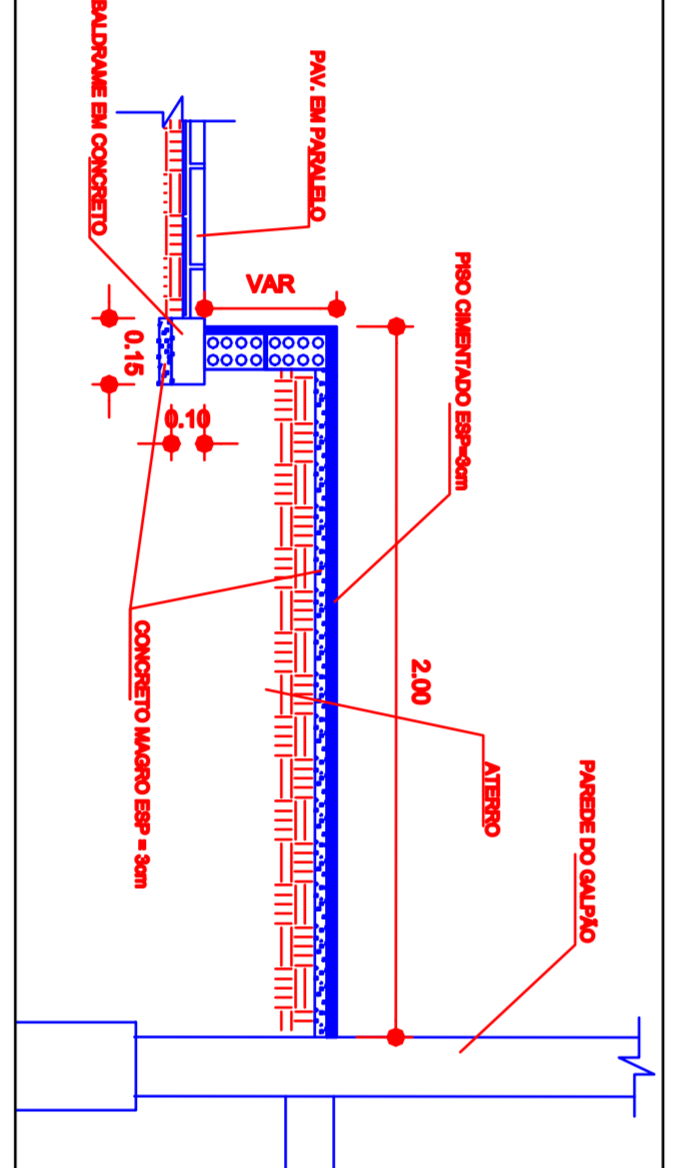
DET. CALÇADA ESC:1/25
