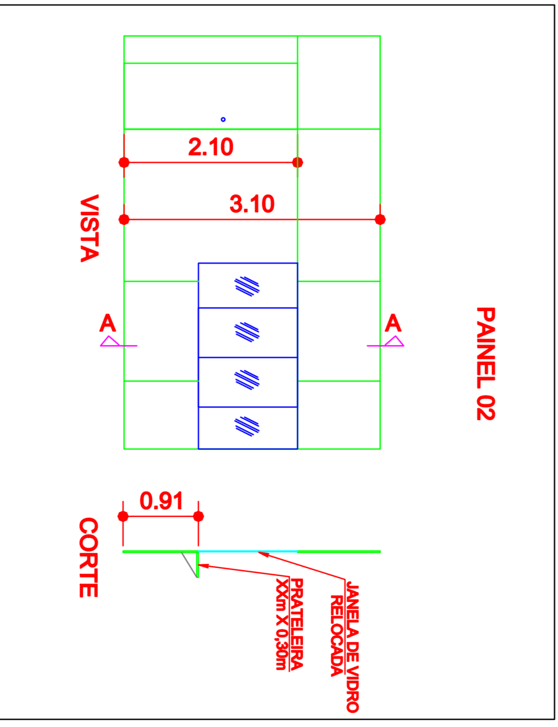
DET 02 ESC:1/100
