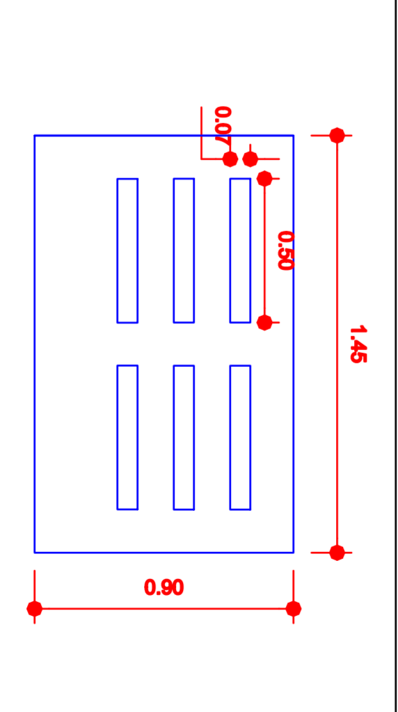
DET. TAMPA DRENAGEM ESC:1/20
